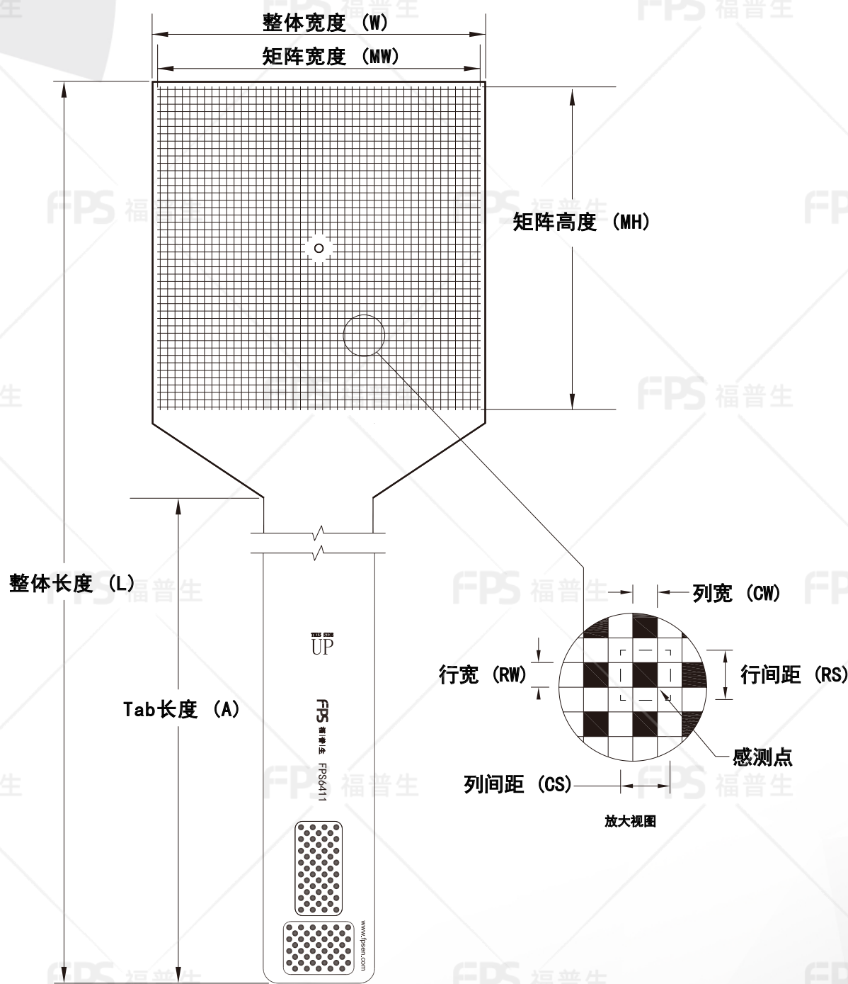
外形尺寸
