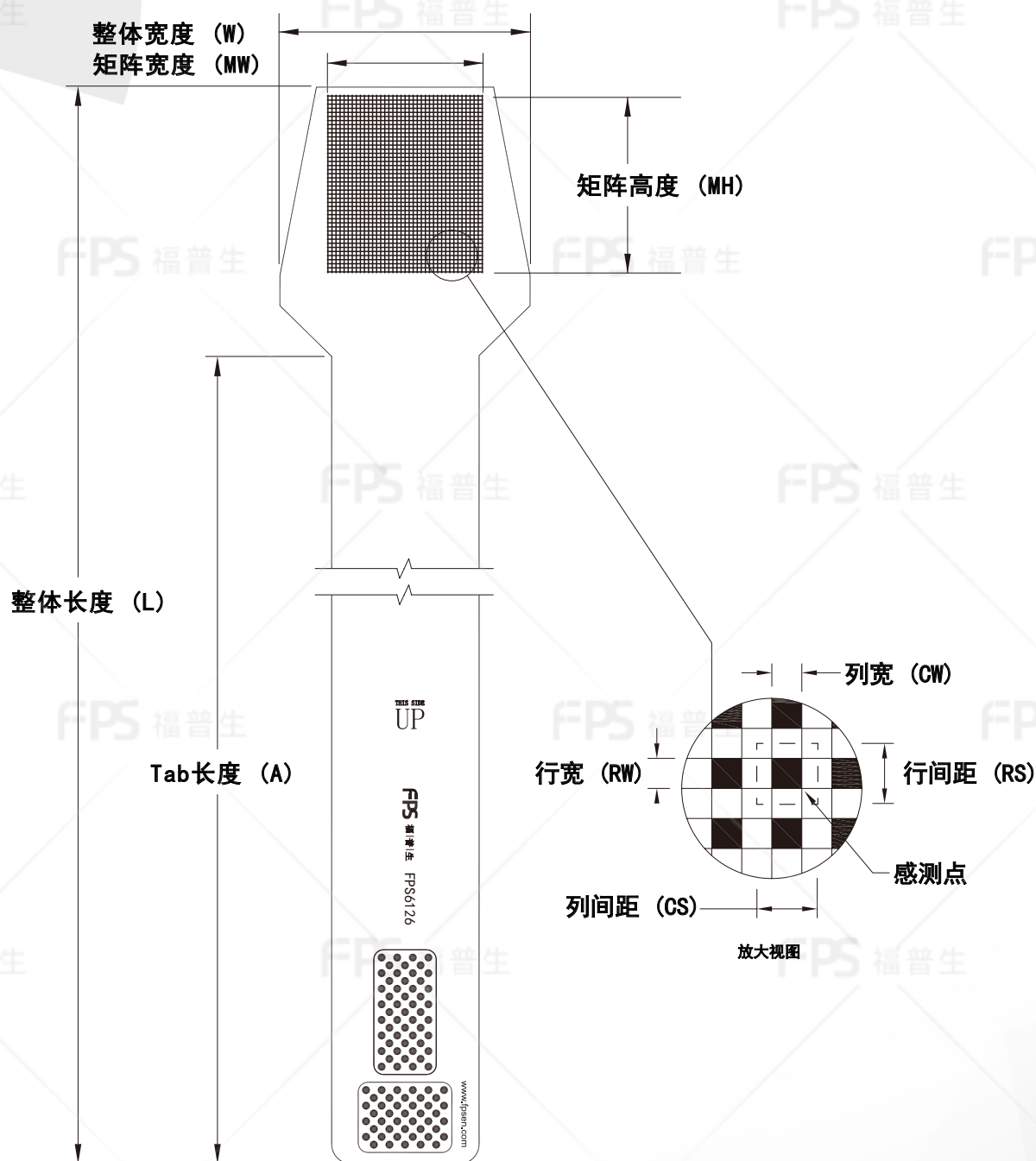
外形尺寸
