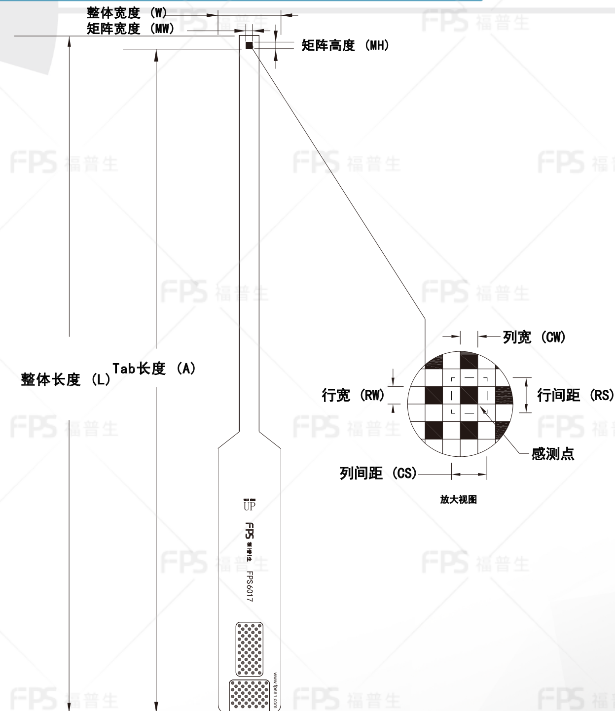
传感区参数
