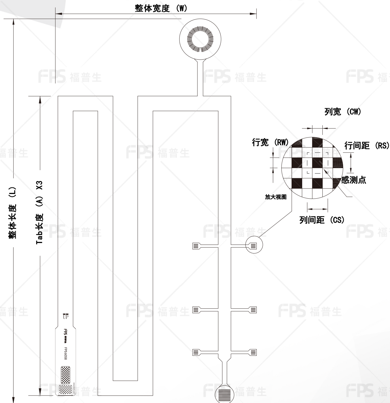
外形尺寸
