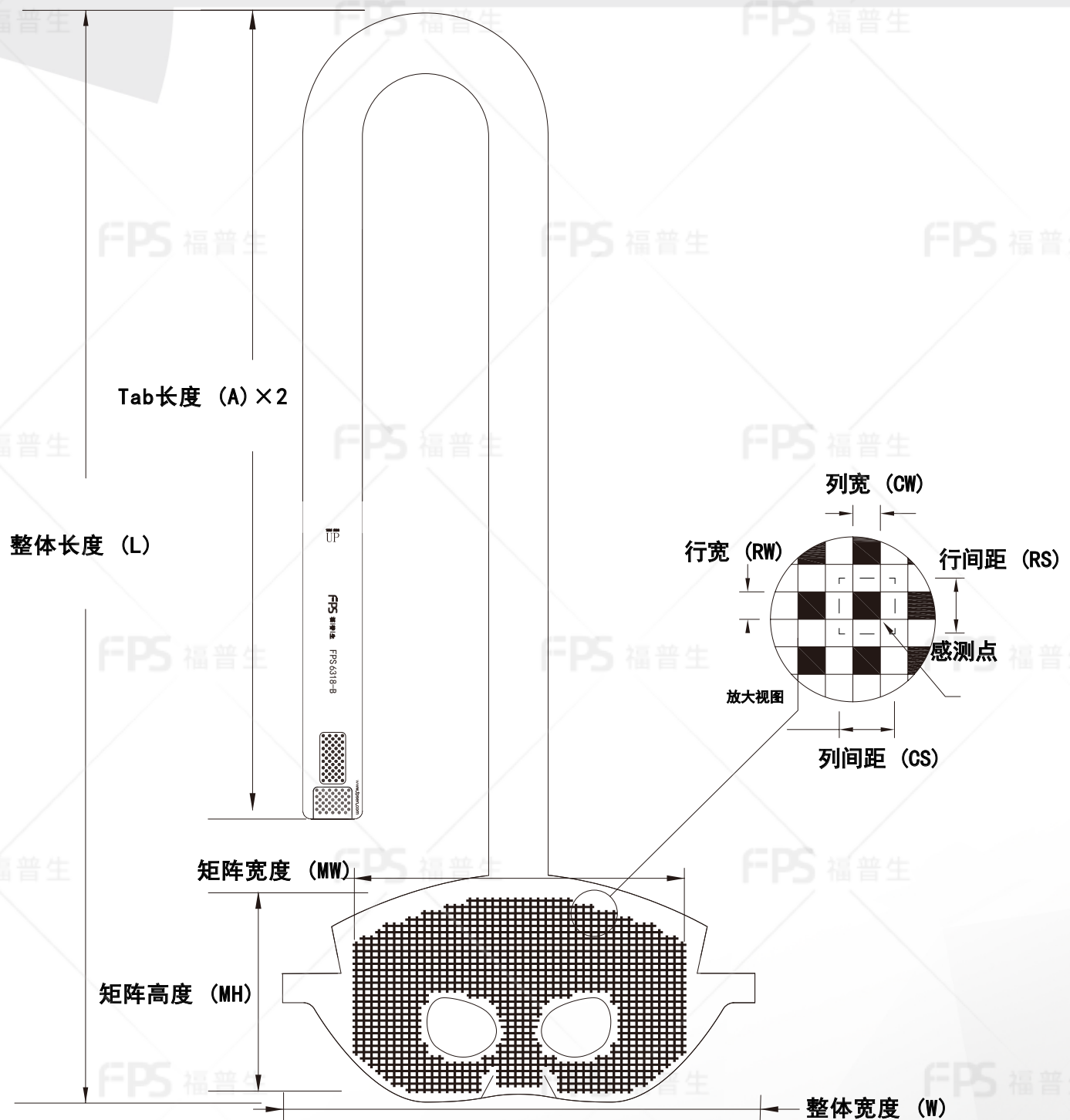
外形尺寸
