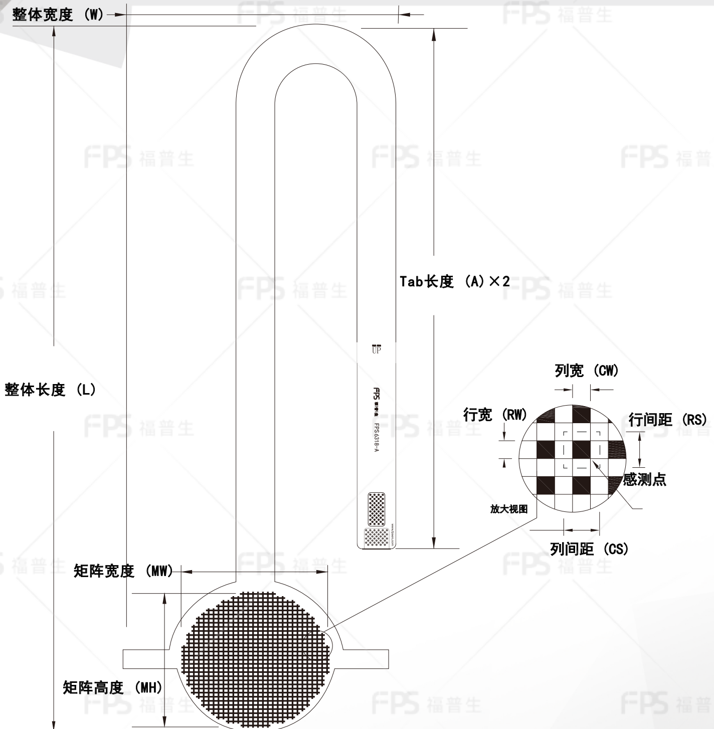
外形尺寸
