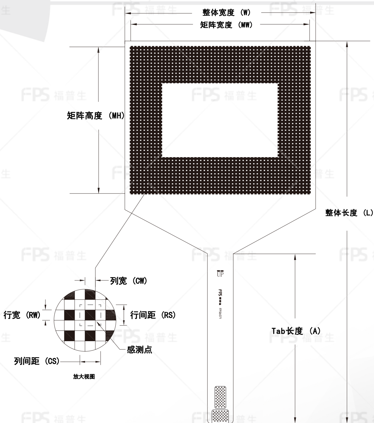
外形尺寸
