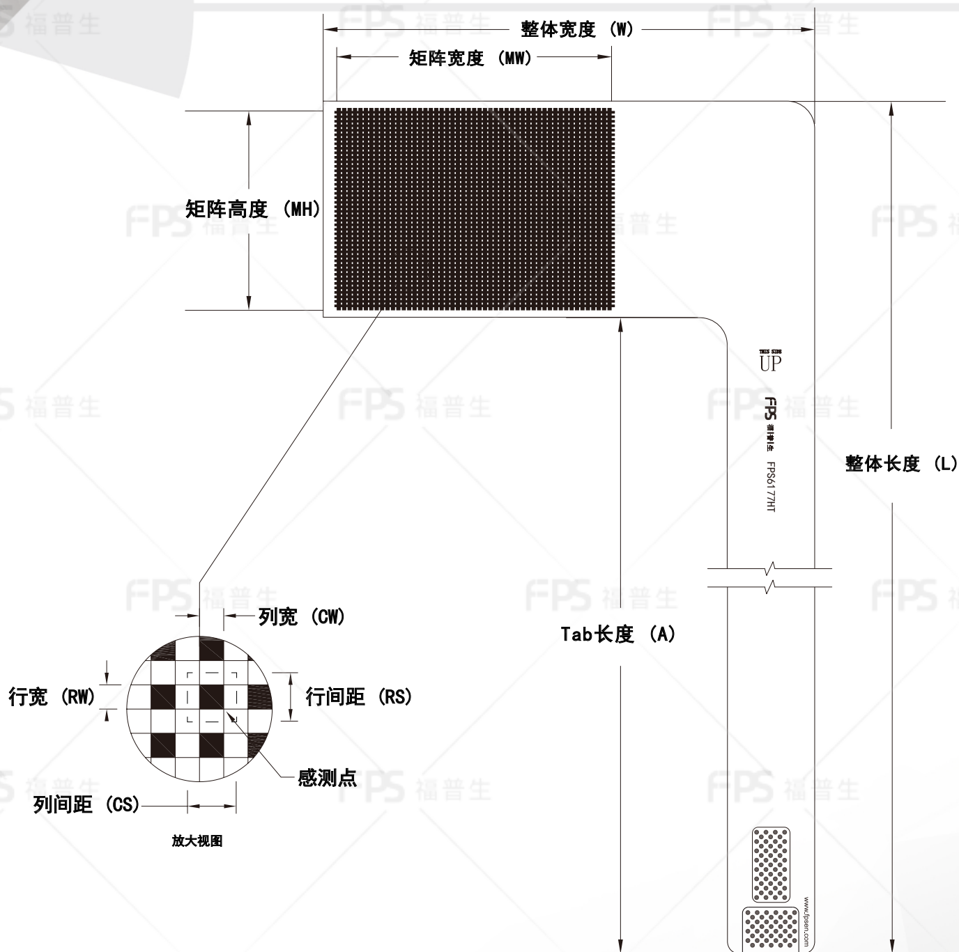
外形尺寸
