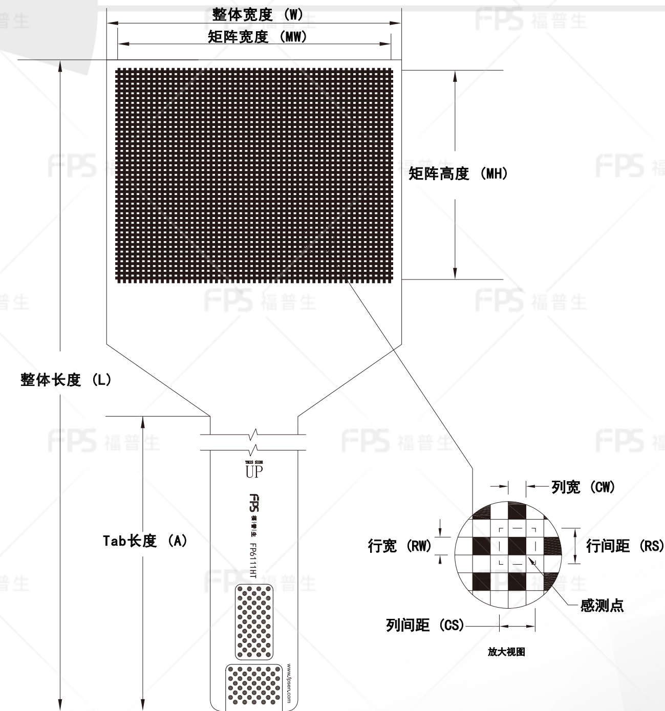
外形尺寸
