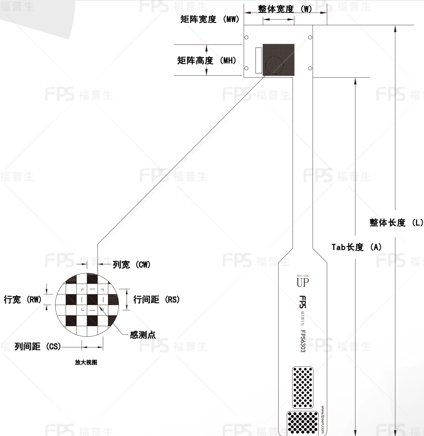
外形尺寸
