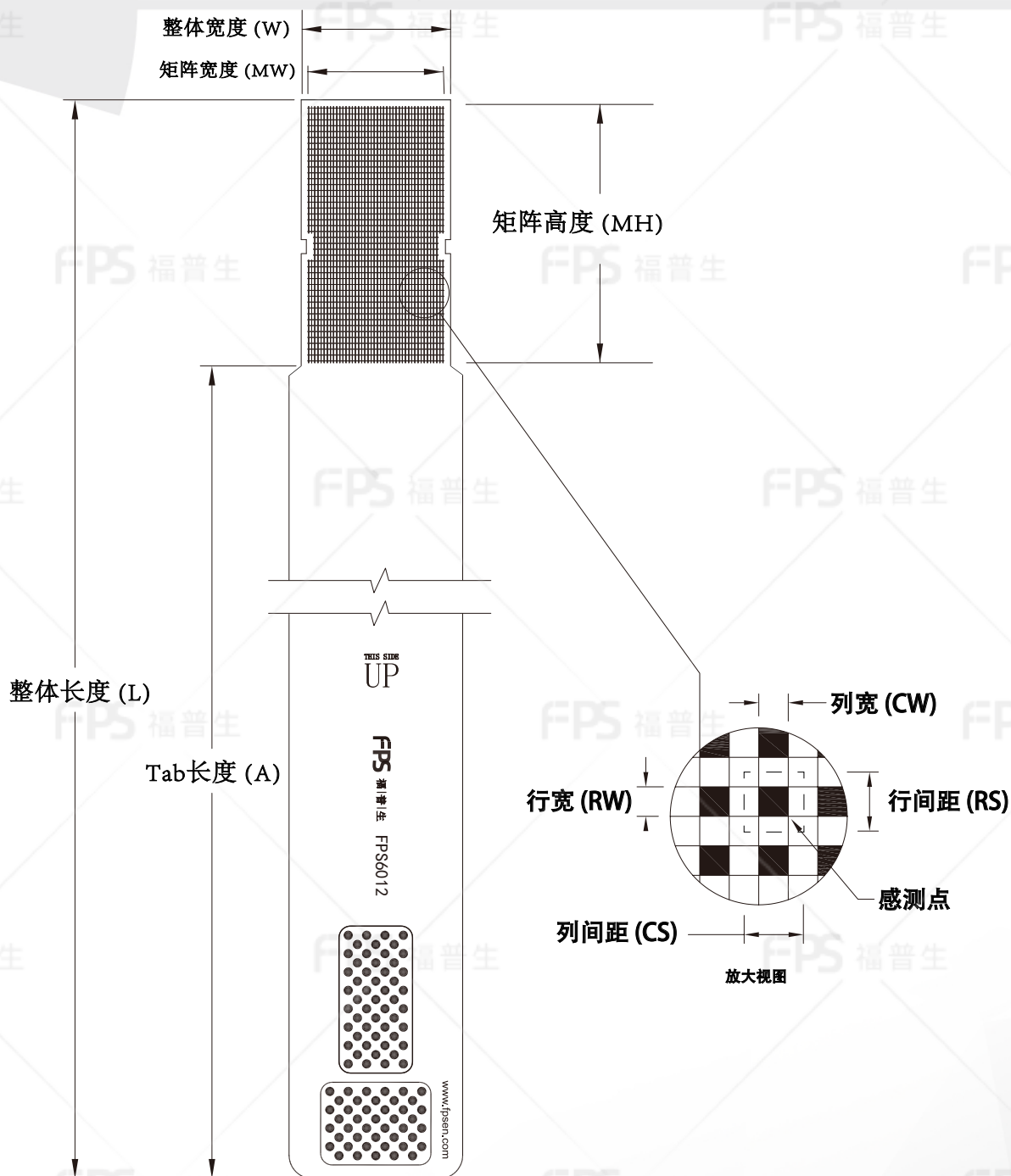
外形尺寸
