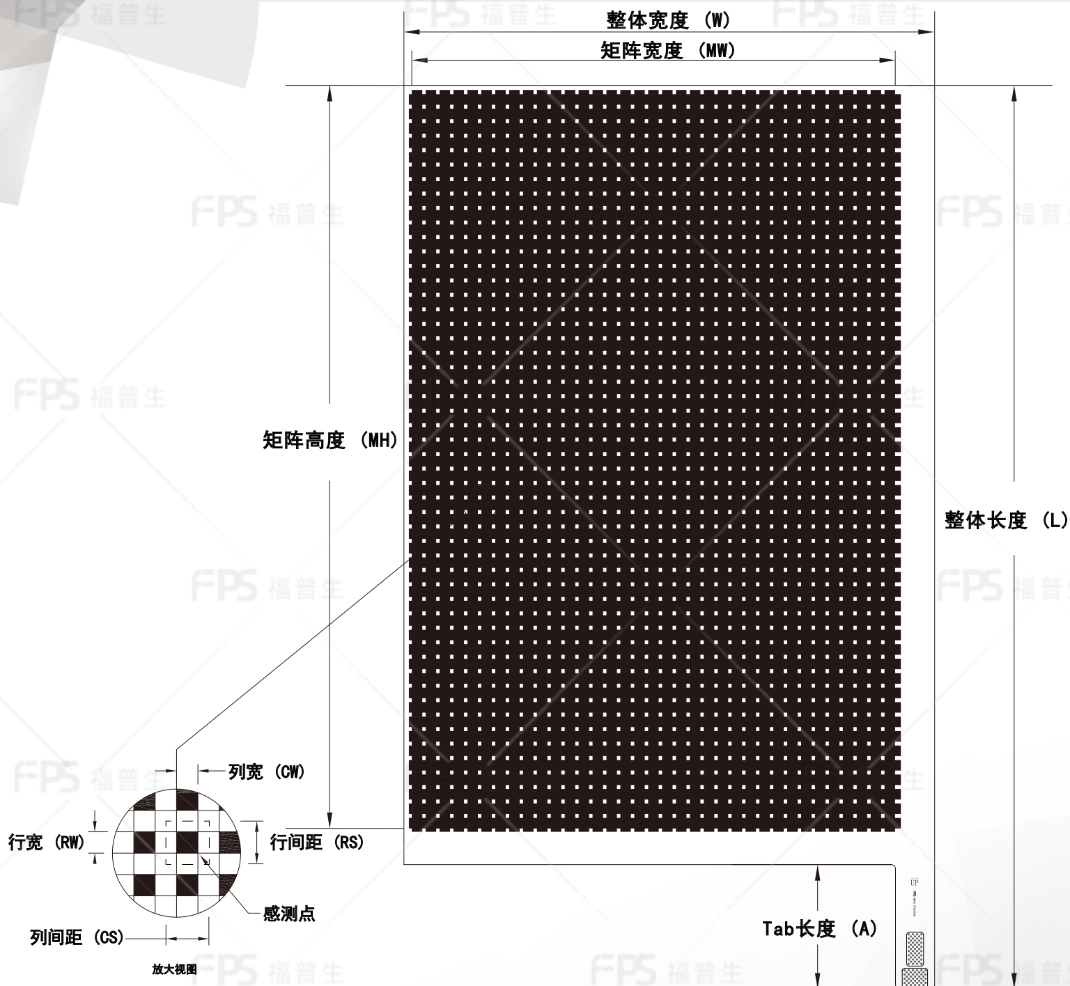
外形尺寸
