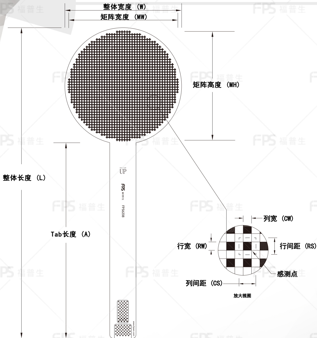
外形尺寸
