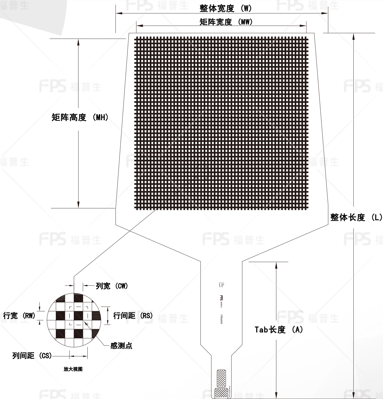
外形尺寸
