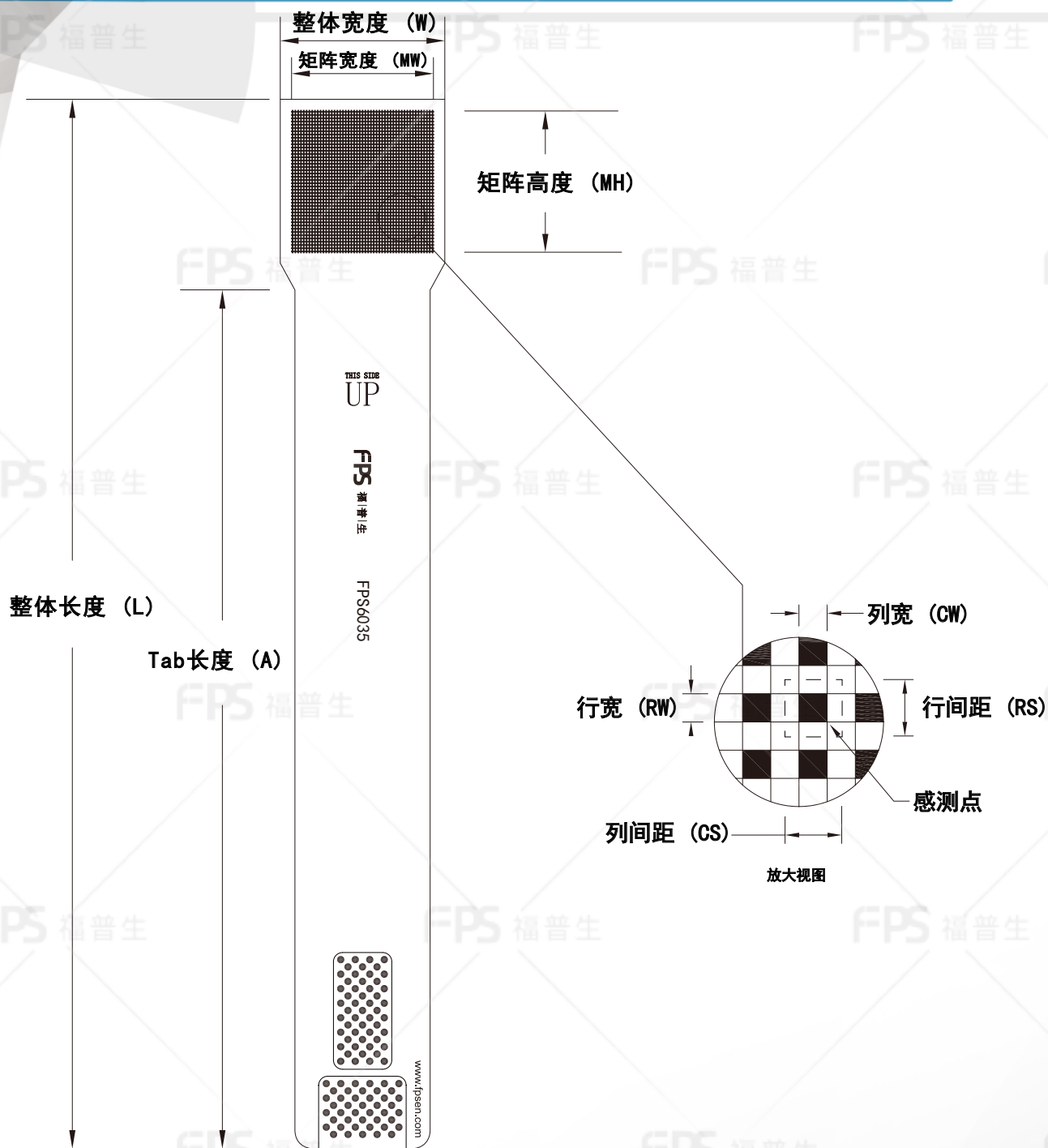
外形尺寸
