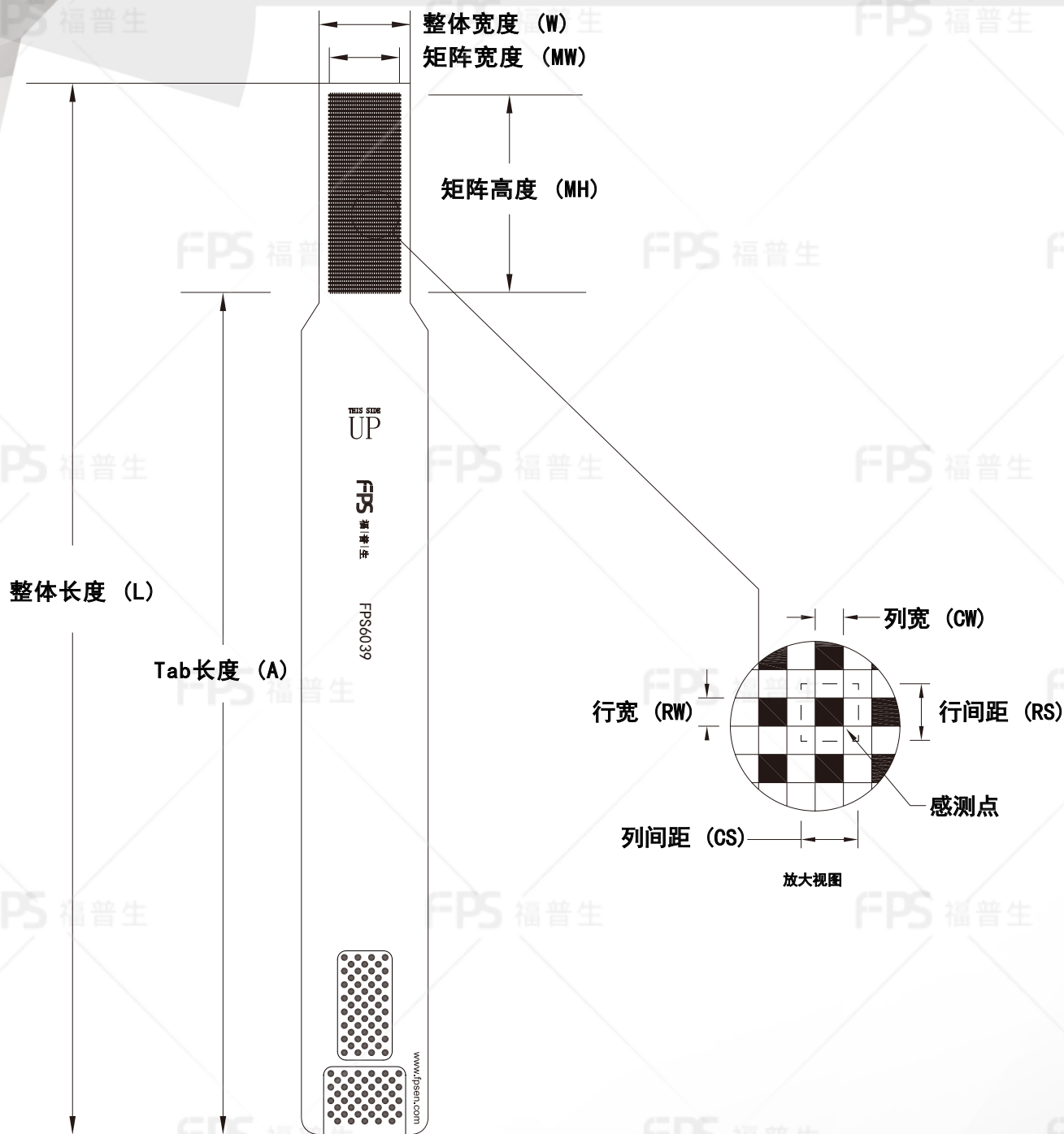
外形尺寸
