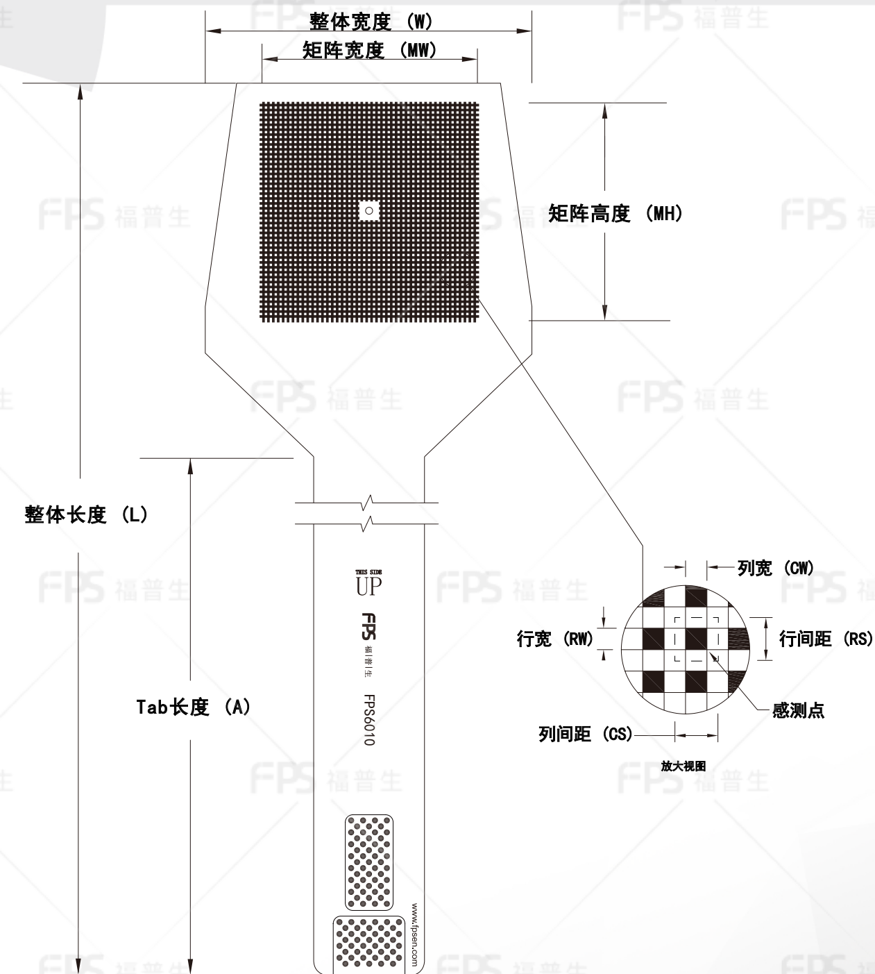
外形尺寸
