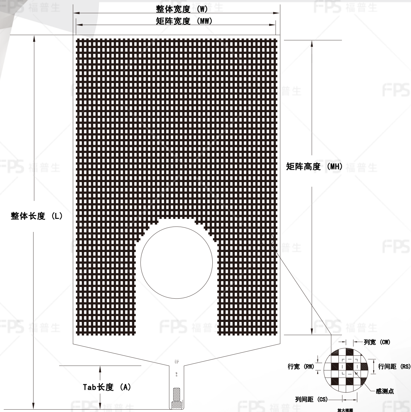
外形尺寸
