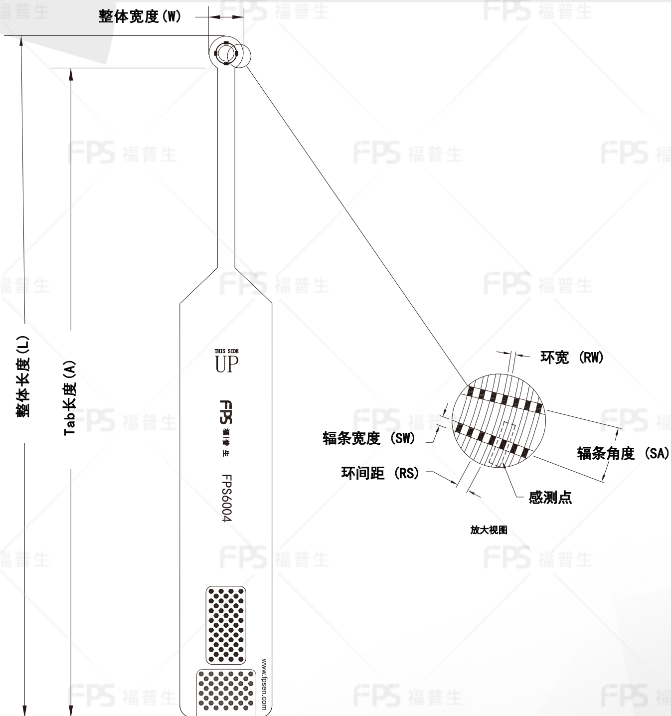
外形尺寸
