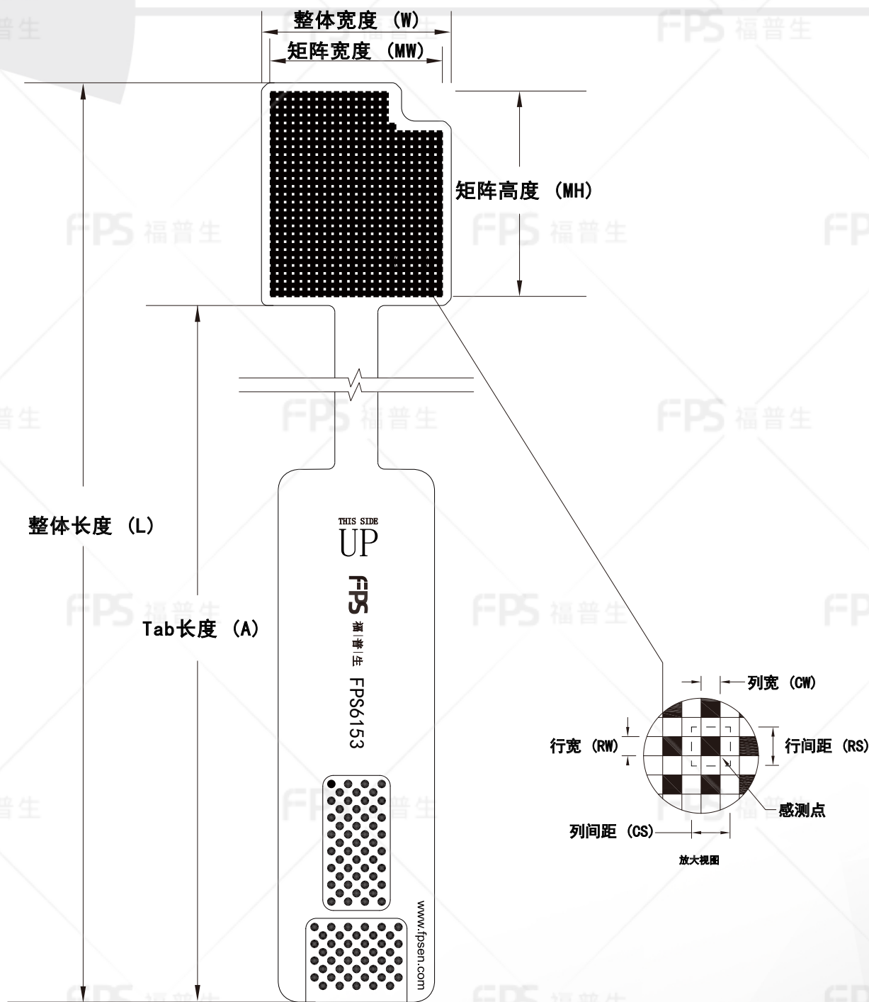
外形尺寸
