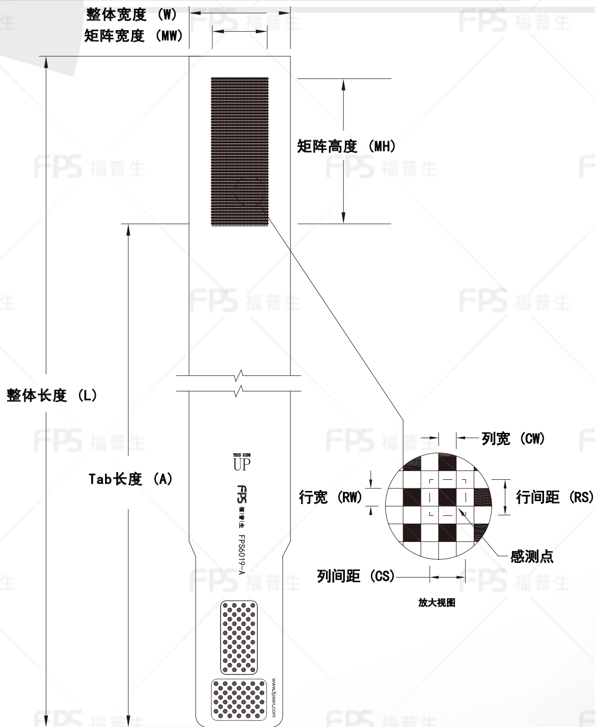
外形尺寸
