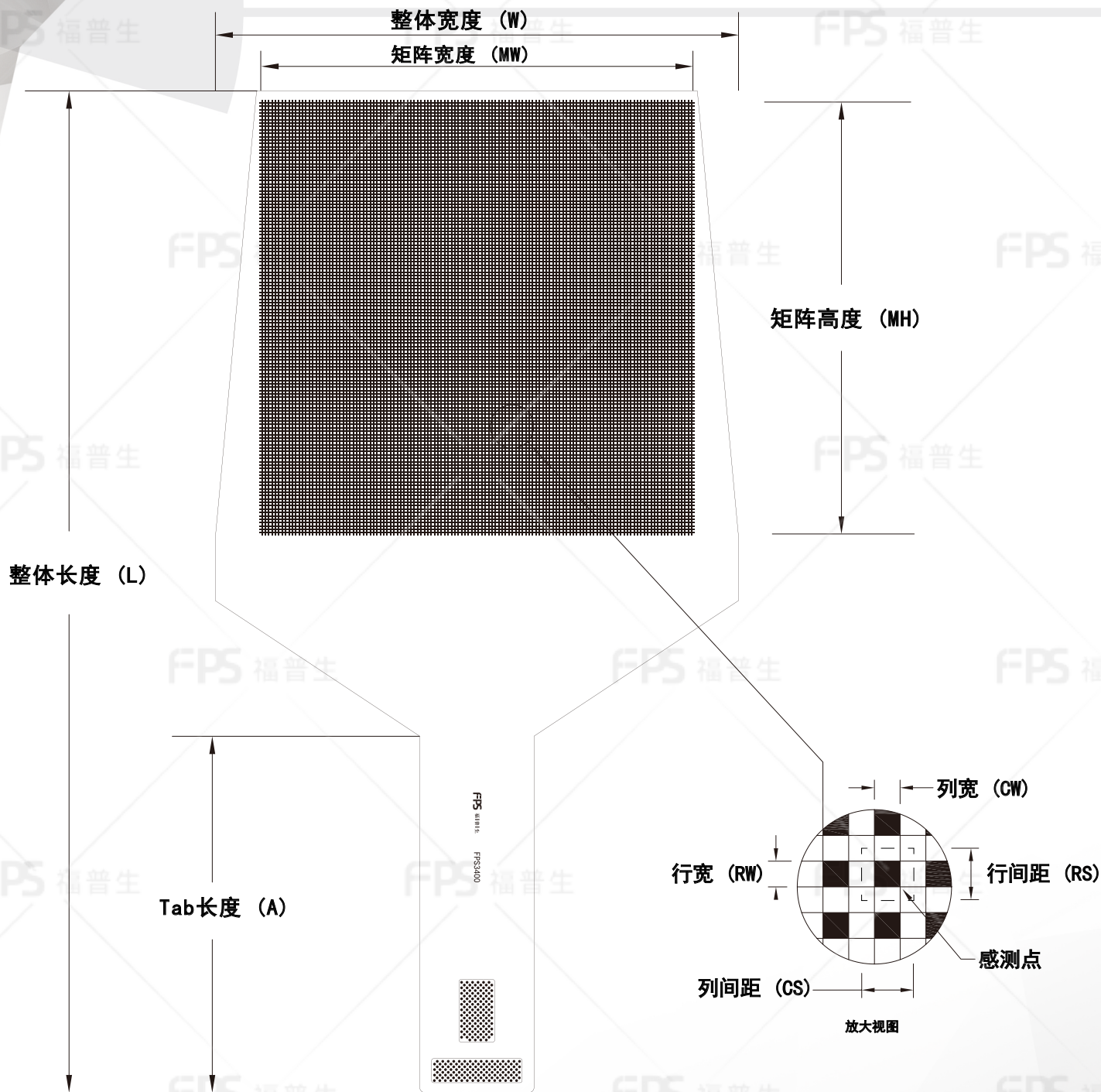
外形尺寸
