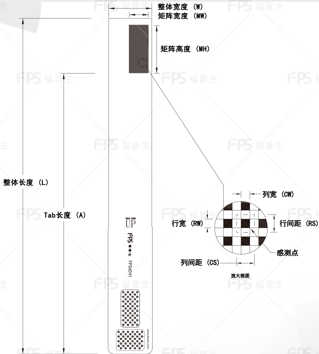
外形尺寸
