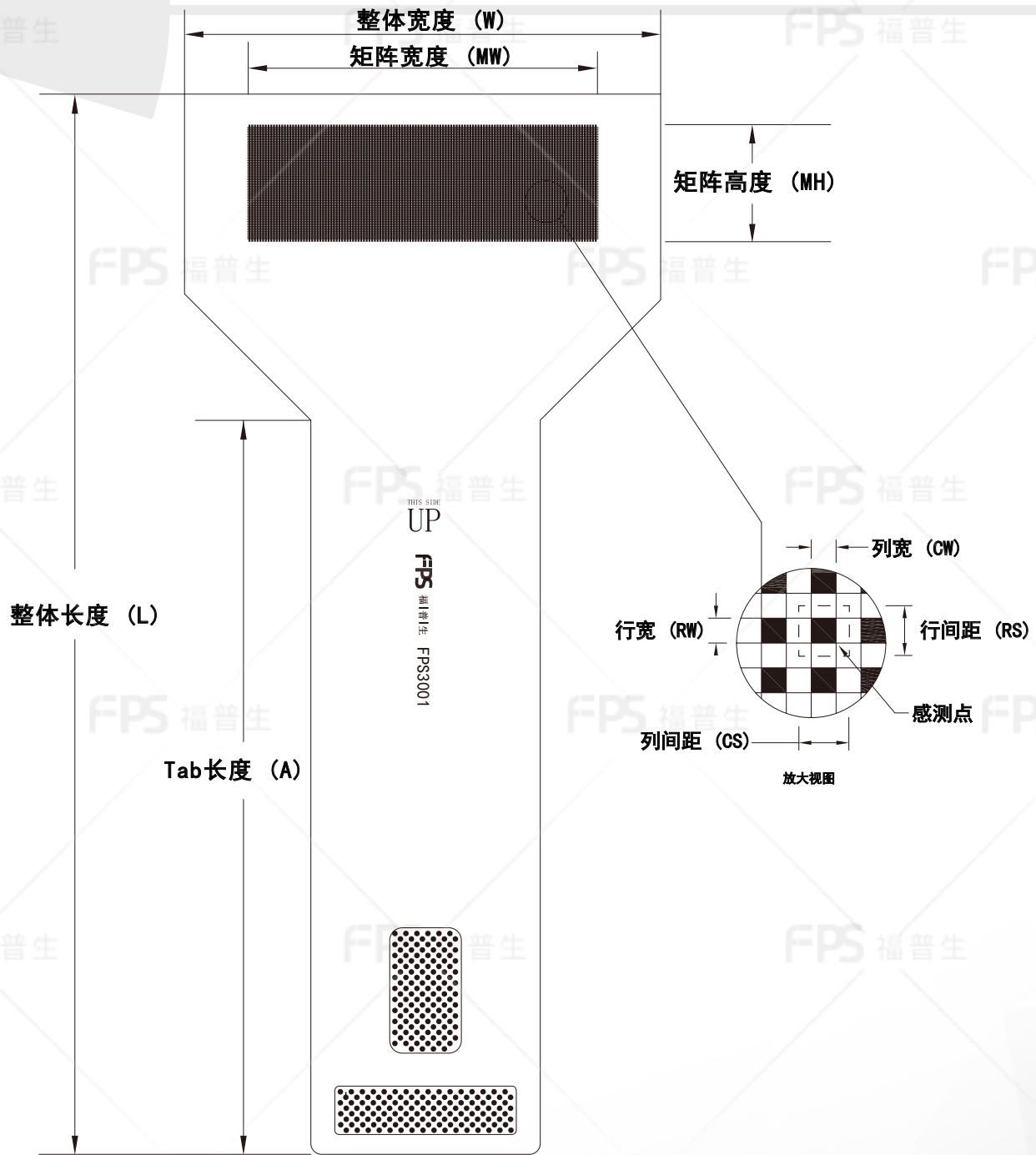
外形尺寸
