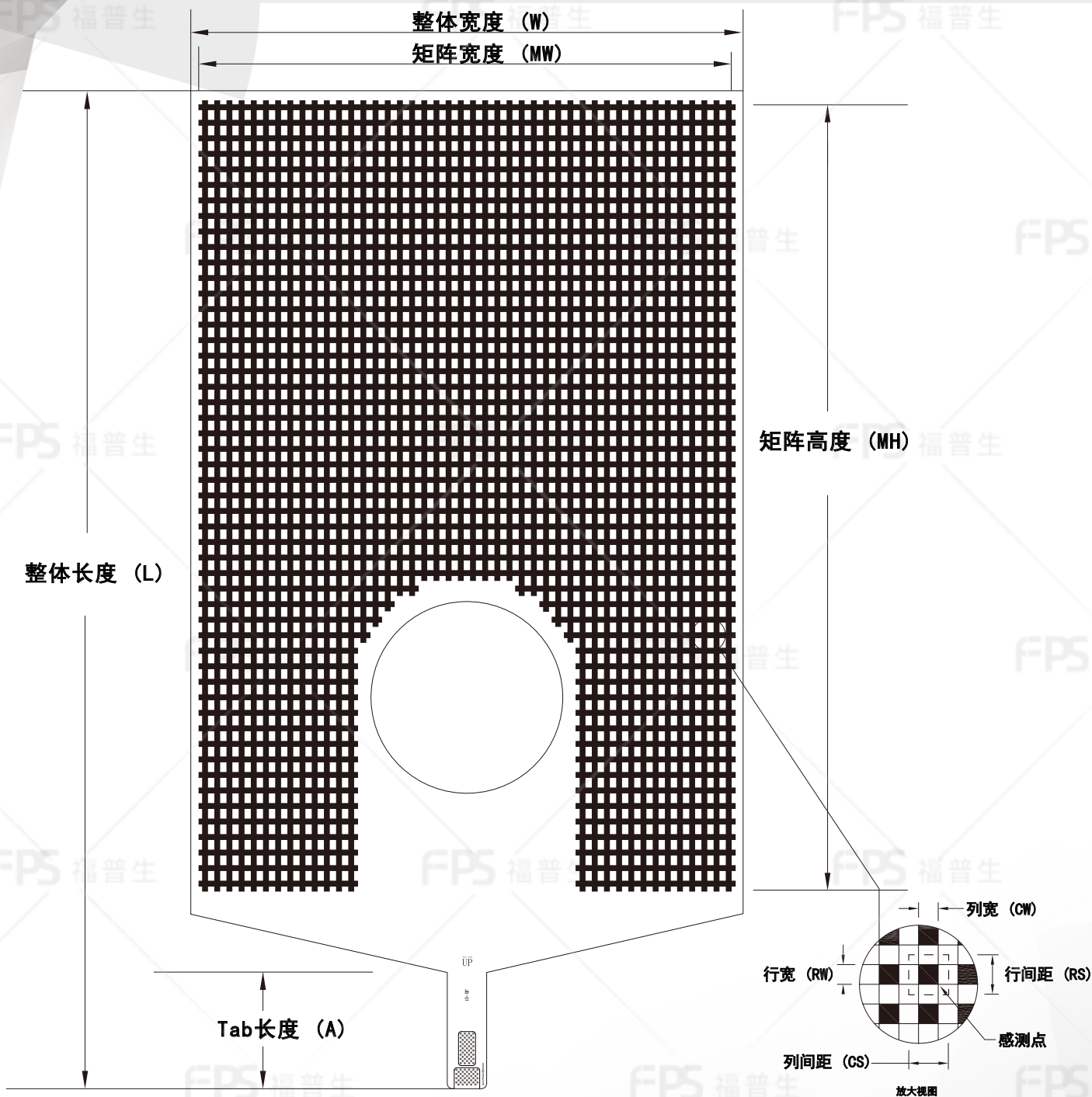
外形尺寸
