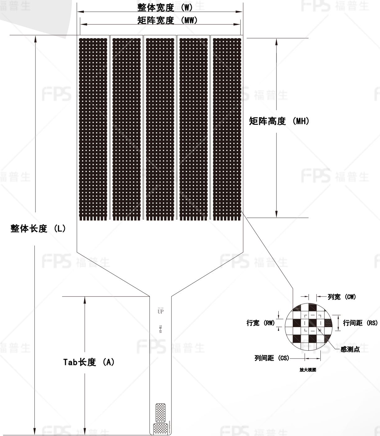
外形尺寸
