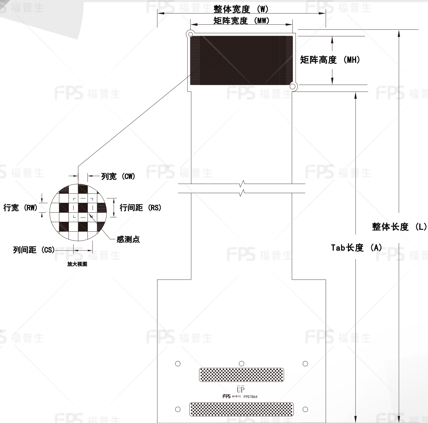
外形尺寸
