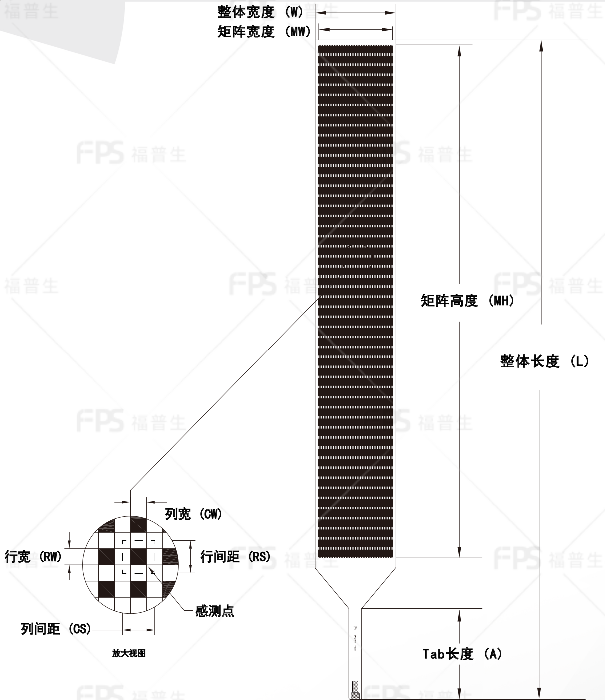
外形尺寸
