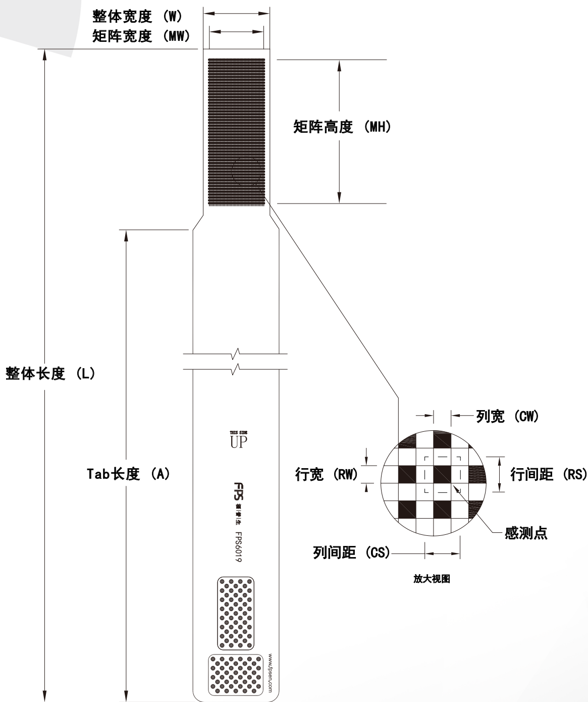
外形尺寸
