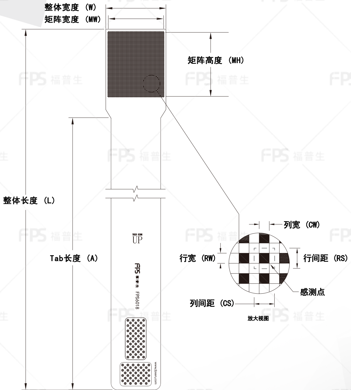
外形尺寸
