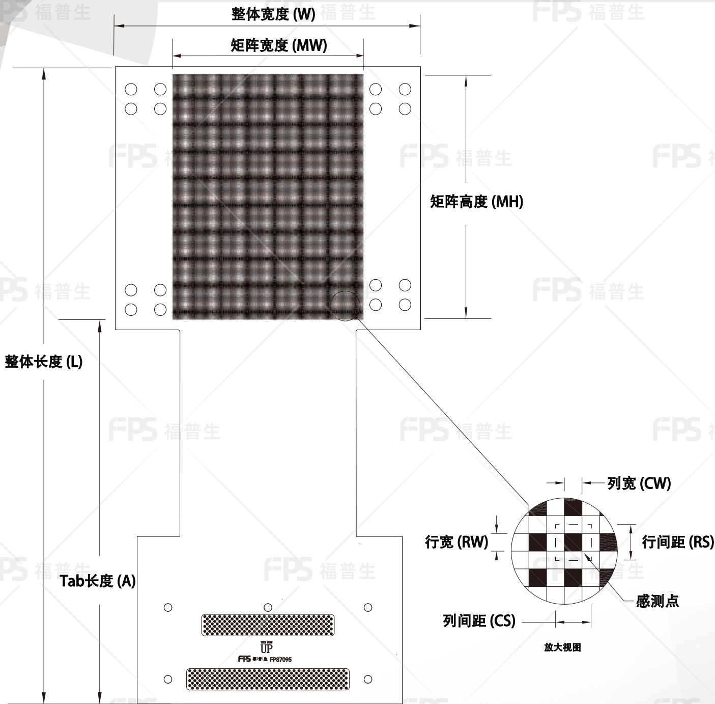
外形尺寸
