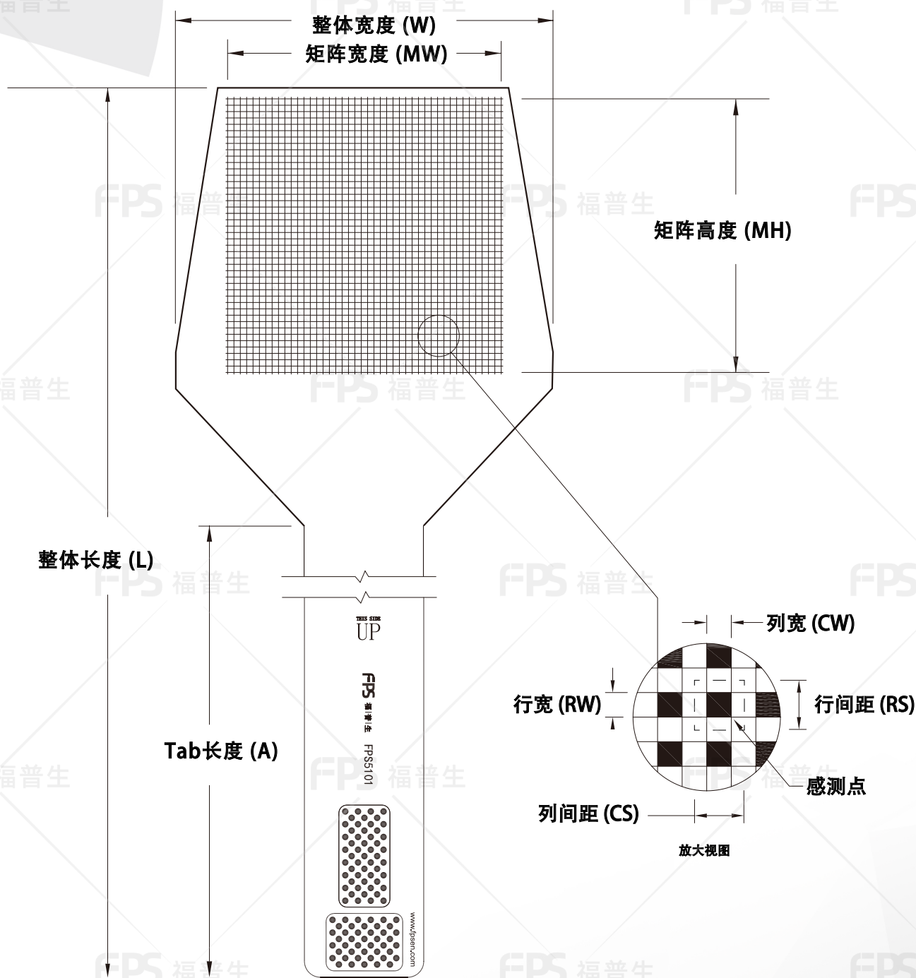
外形尺寸
