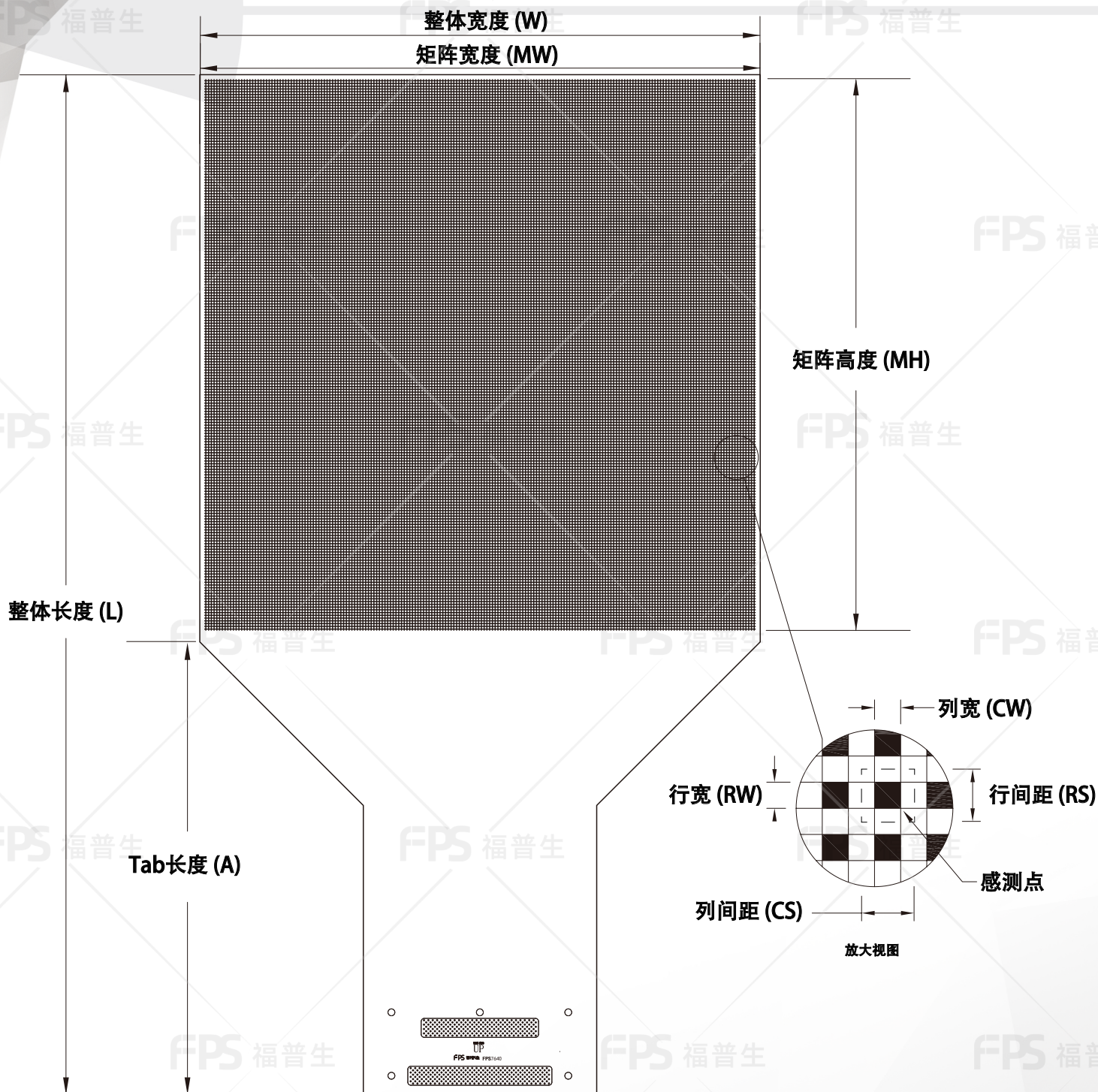
外形尺寸
