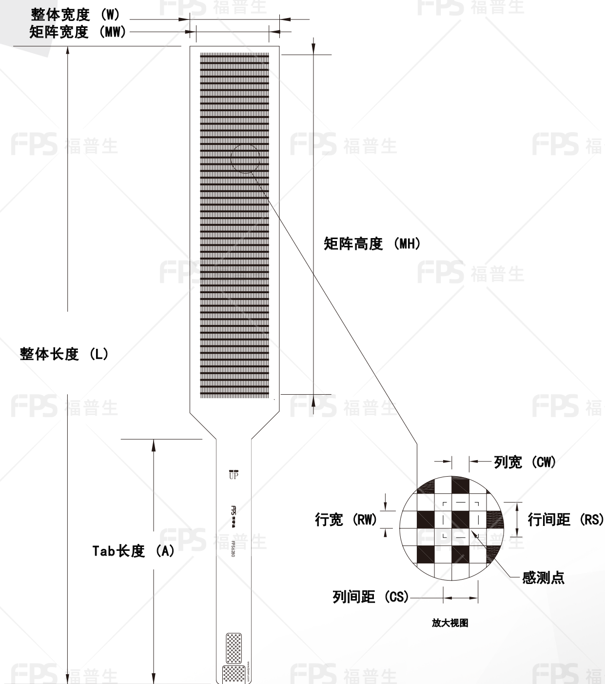
传感区参数
