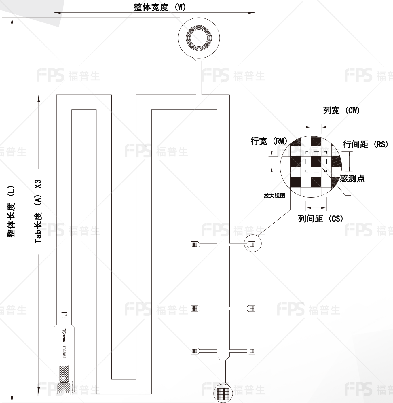
外形尺寸
