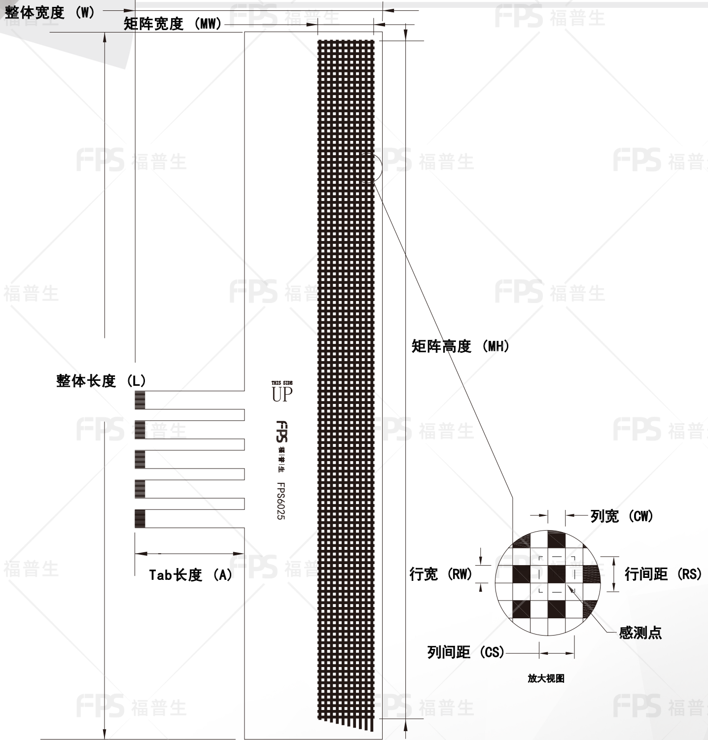
外形尺寸
