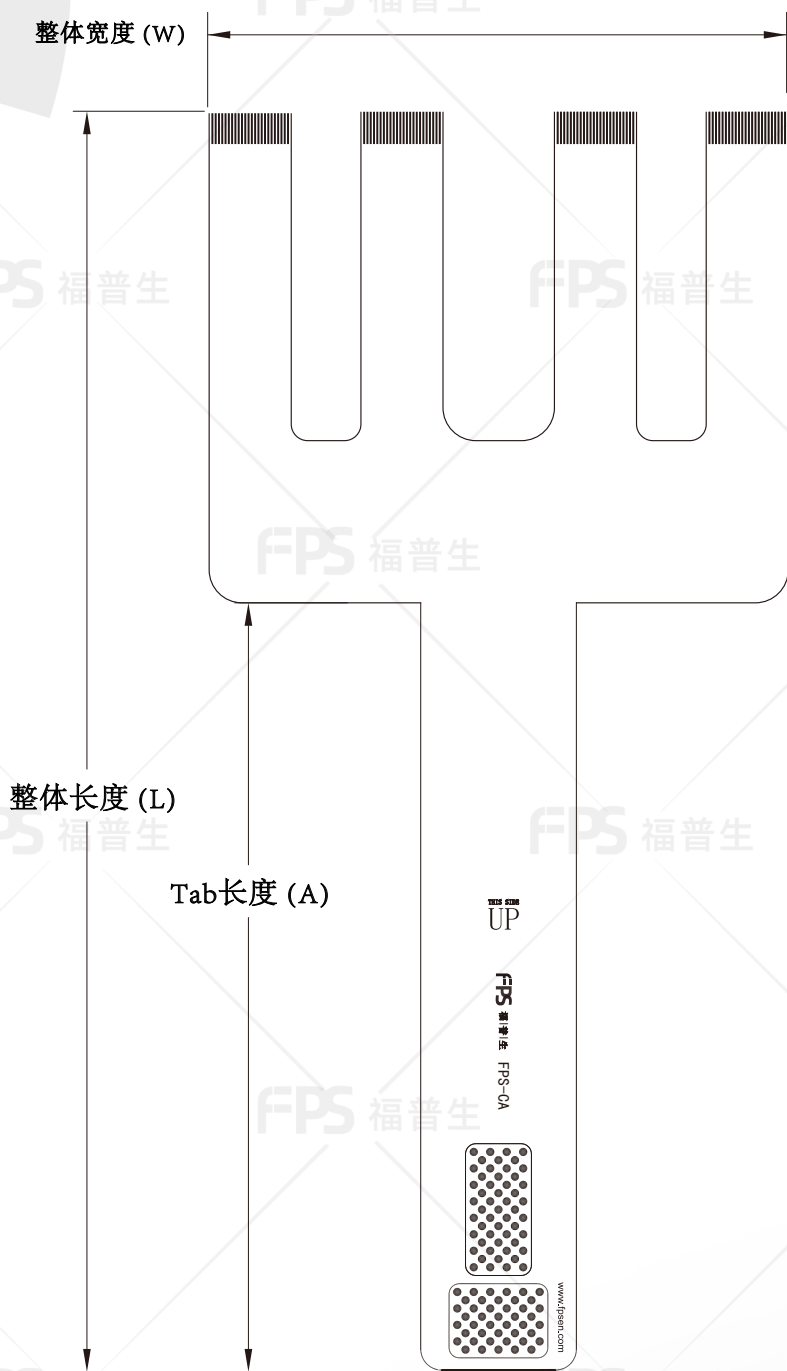
传感区参数
