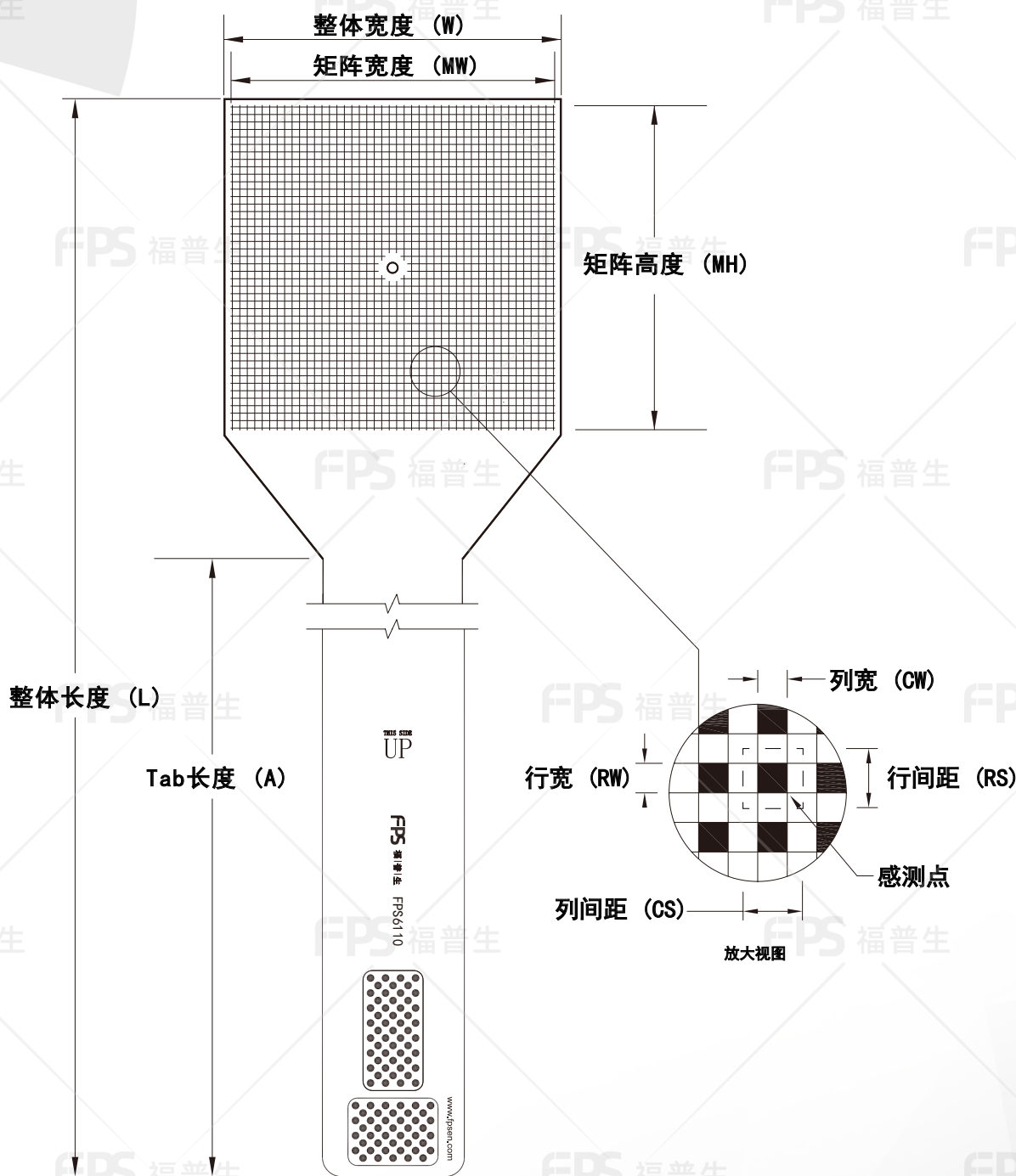
外形尺寸
