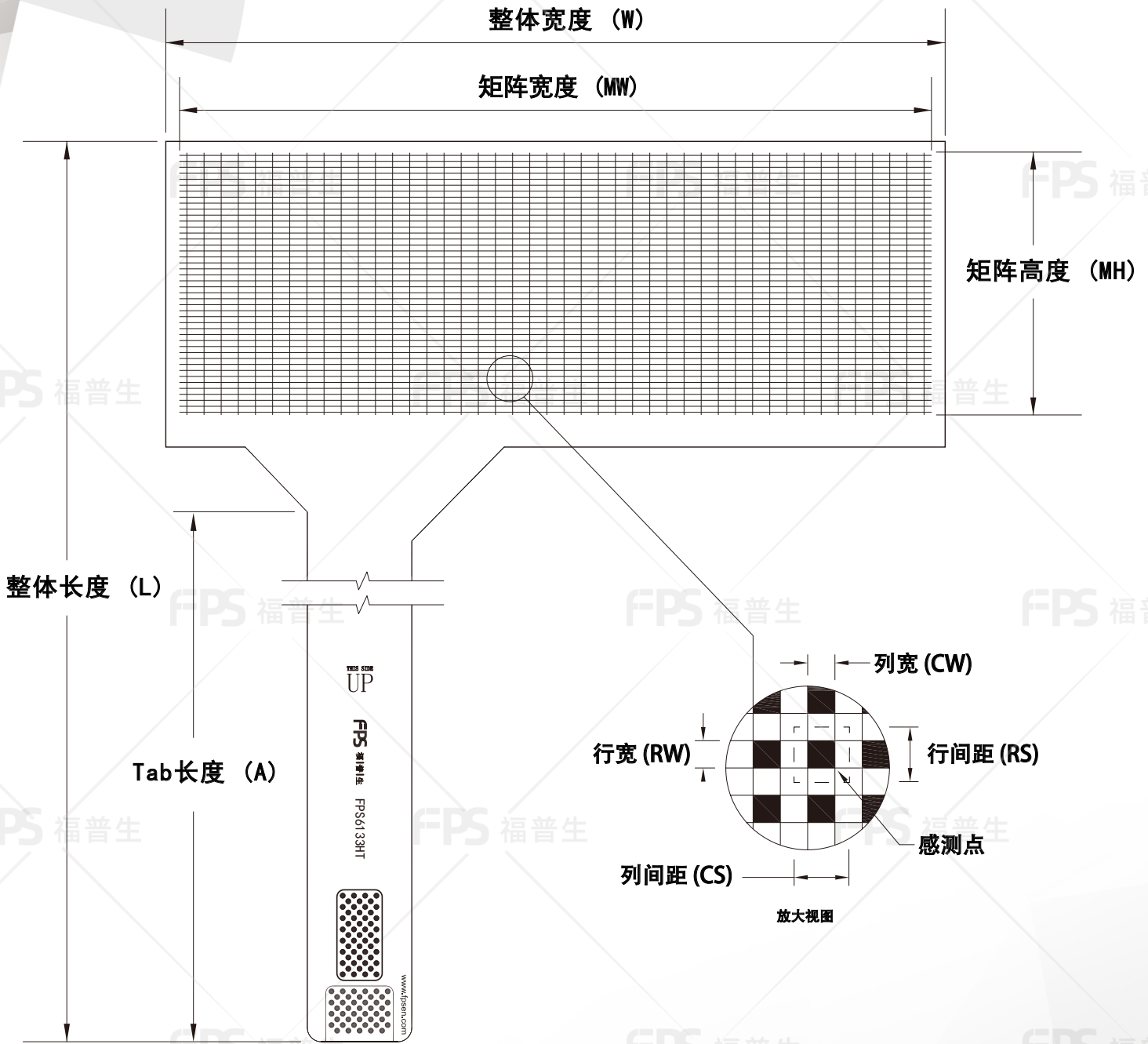
外形尺寸
