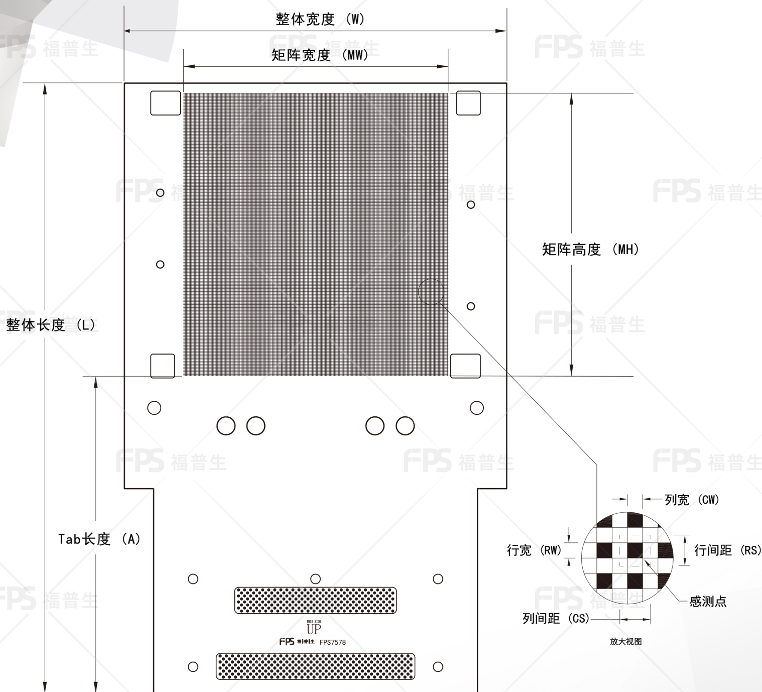
外形尺寸
