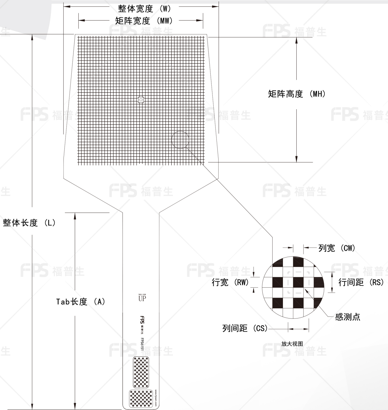
外形尺寸
