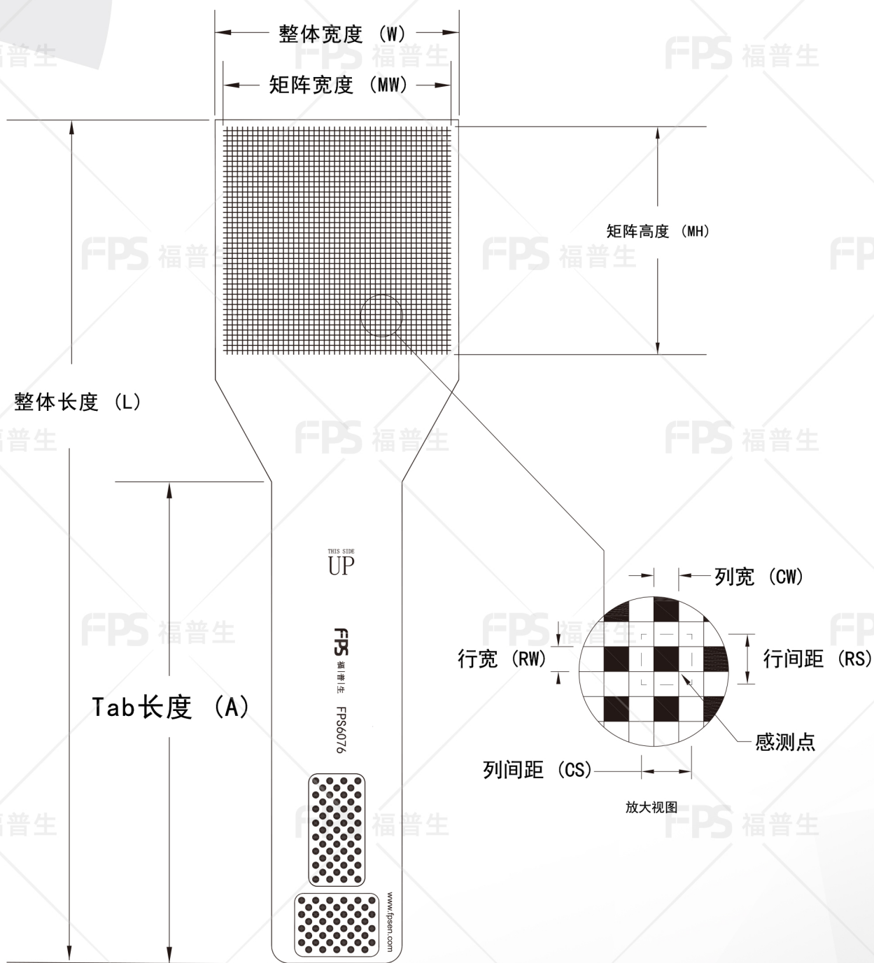
外形尺寸
